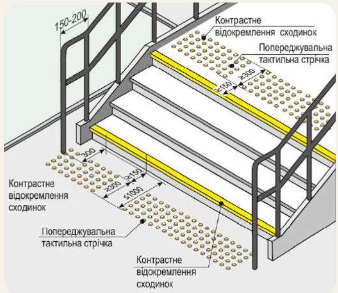
Рисунок 1.14. Облаштування сходінок
