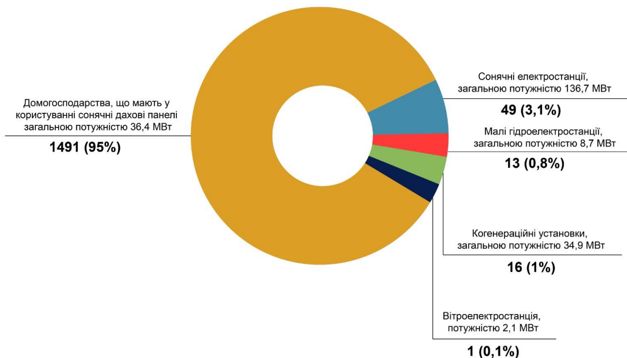
Мал. 7 Об'єкти розподіленої генерації, що діють в області
